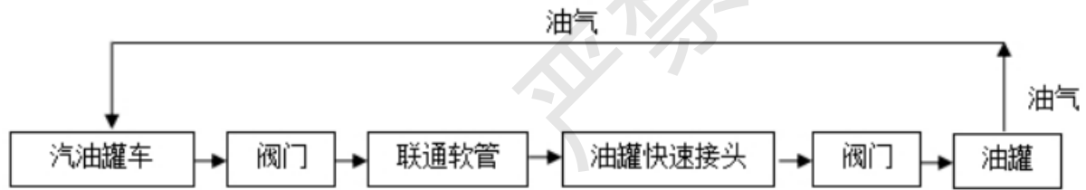
卸油工艺流程方块图
