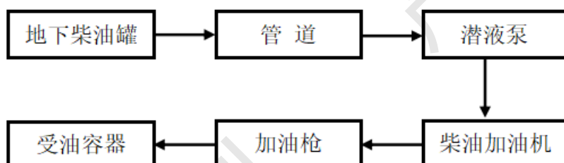
图 2-3 加油工艺流程图
