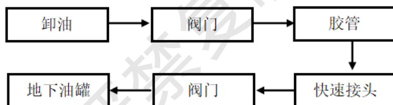
图 2-2 卸油工艺流程
