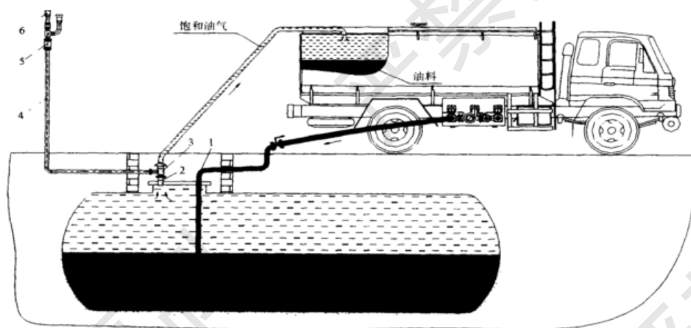
图 2-6 第一阶段油气回收系统示意图
